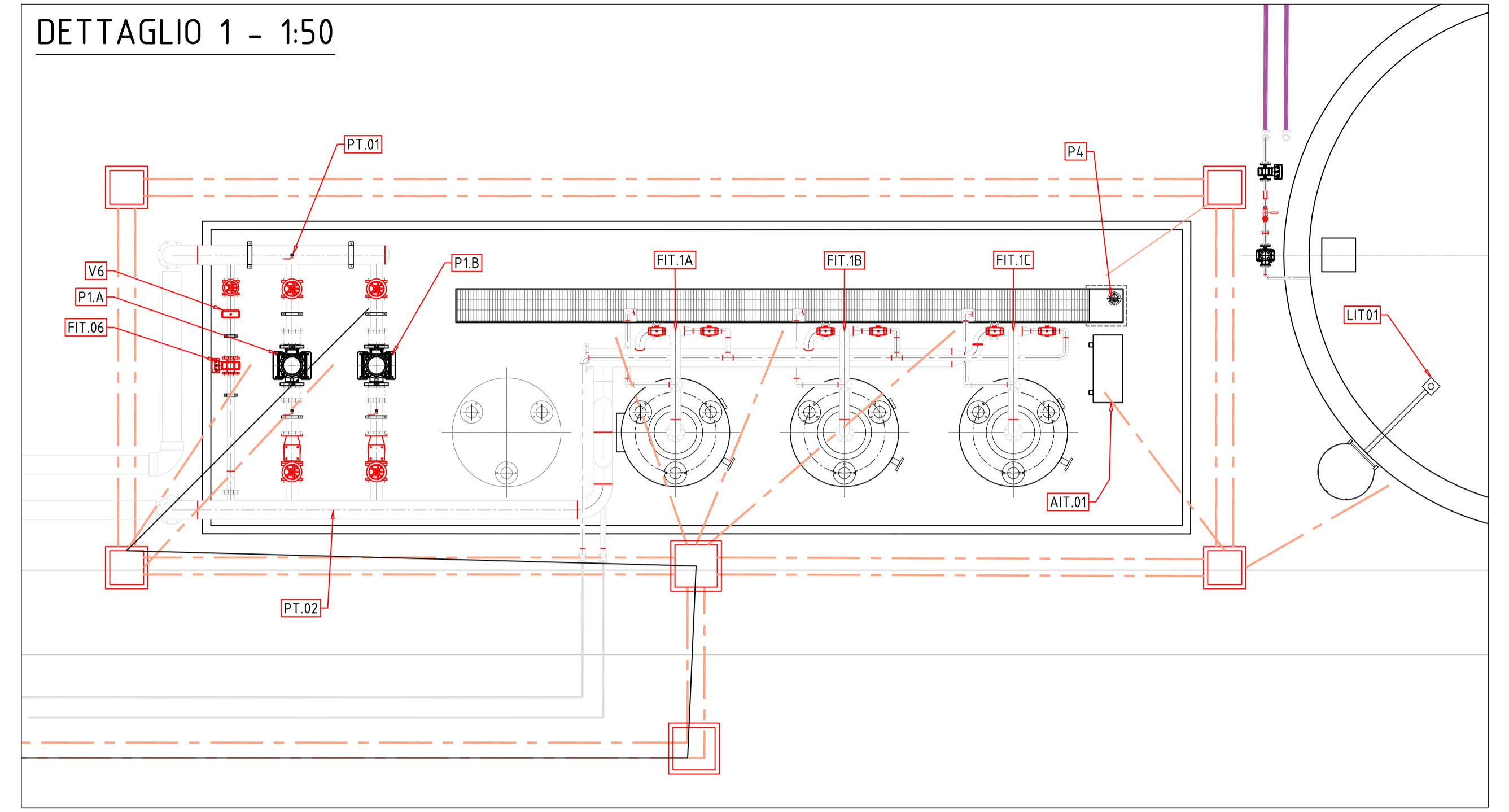
DETTAGLIO 2 - 1:50
